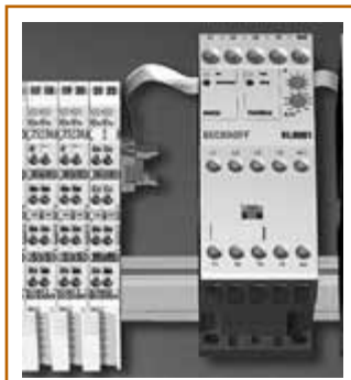
Рис. 2. Модуль-адаптер KL8001, построенный на основе модулей измерения потребляемой мощности (KL3403), обладает также функциями коммутации
