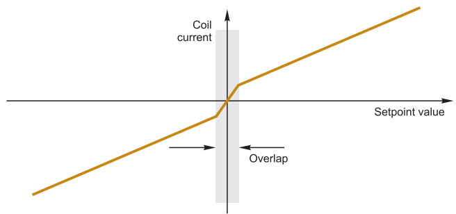
Рис. 3. Характеристическая кривая тока обмотки в клапане Эффект перекрытия предотвращает линейный ход вблизи нулевой точки, при этом малое изменение уставки не влияет на изменение расхода жидкости. Путем подачи в систему тока постоянного смещения удается добиться более линейного регулирования изменения расхода вблизи нулевой точки. Величина зоны перекрытия является свойством клапана и зависит от его типа
