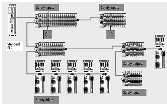
Рис. 2. В рамках проекта по развитию системы модулей для промышленной сети EtherCAT создан простой, эффективный и недорогой контроллер безопасности локального уровня
